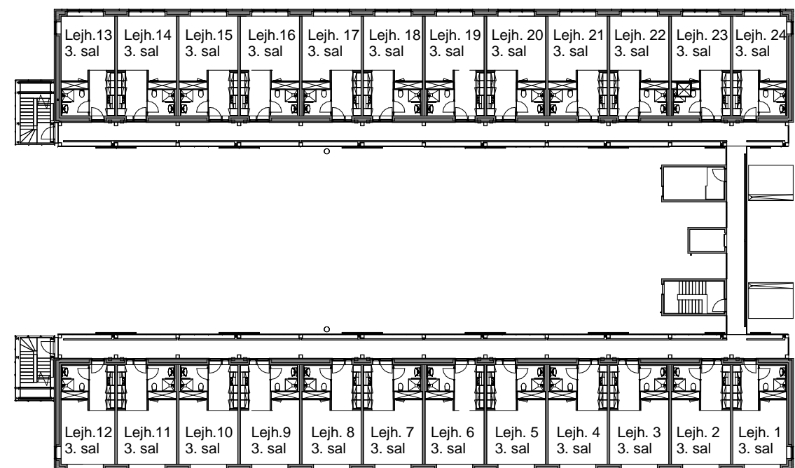
3. SAL
