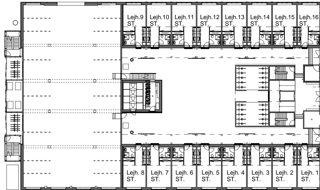
ST.ETAGE
